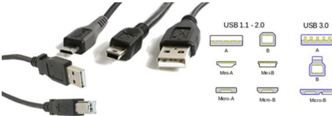
I vari formati dei connettori USB
